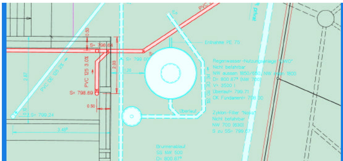
Planausschnitt Regenwasser-Nutzungsanlage
